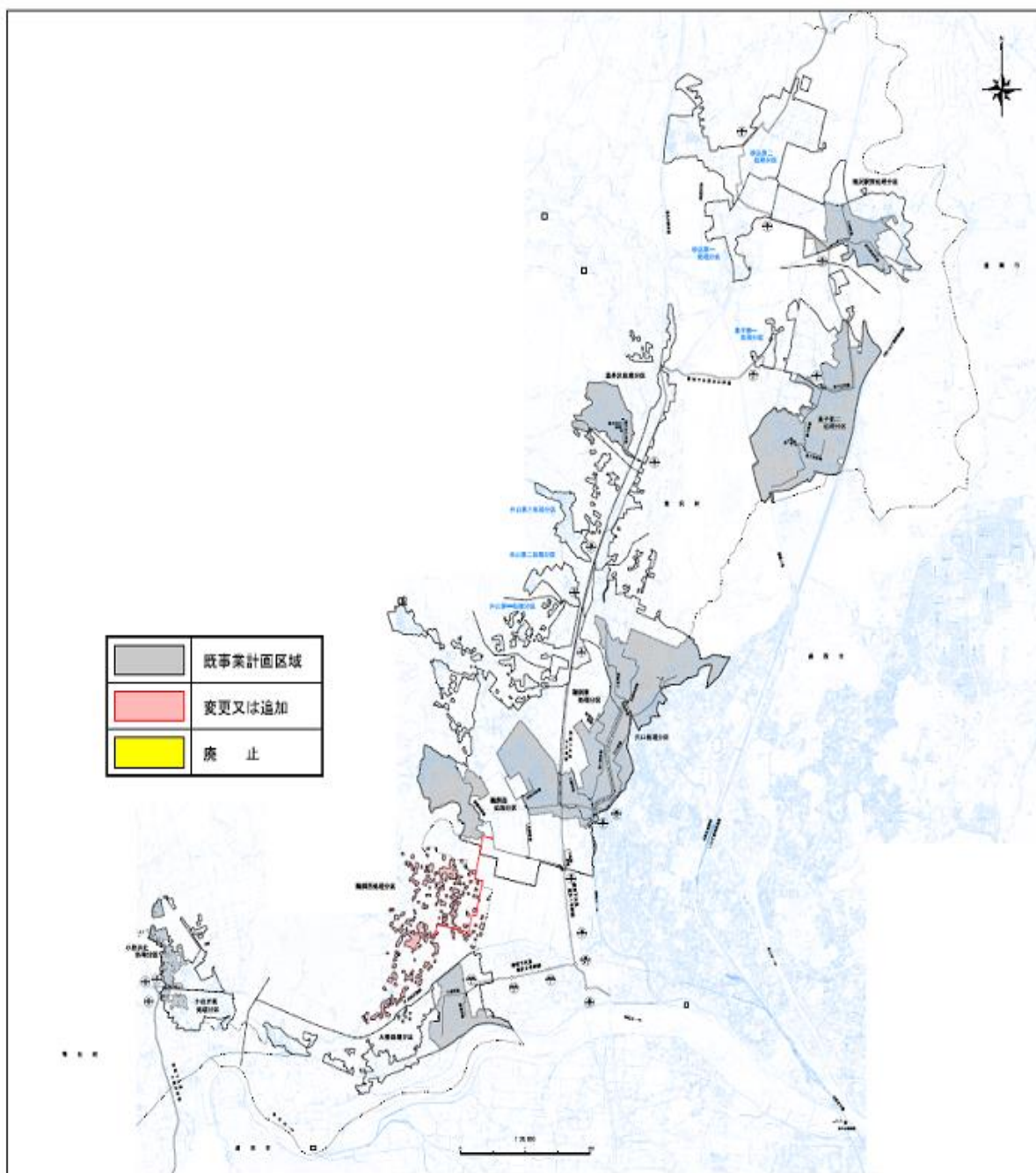
滝沢公共下水道事業計画一般平面図
