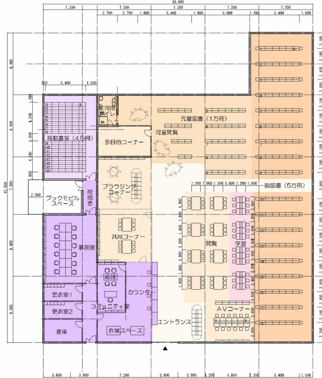
◆CASE-A 書架間寸法2.1m (床面積: 1,255㎡+34㎡=1,289㎡)
