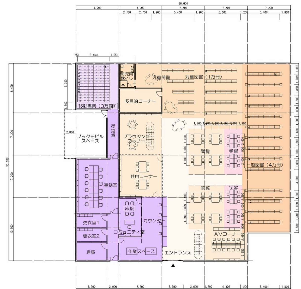
◆CASE-B 書架間寸法1.8m (床面積: 1,131㎡+ブックモビル60㎡=1,191㎡)
