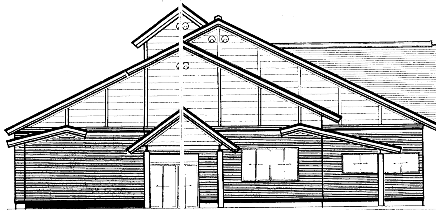
東面
