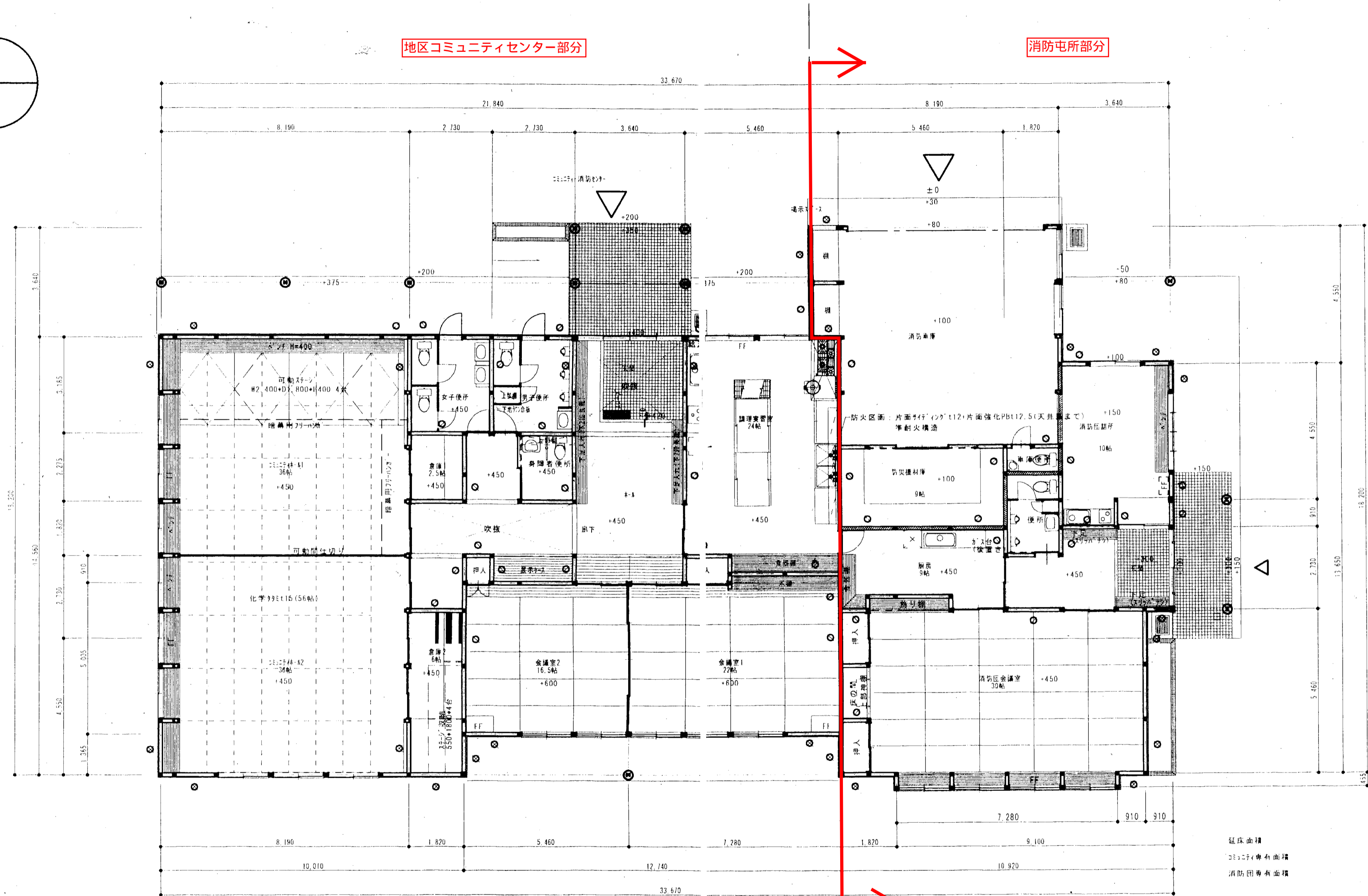
平面図 S=1:100
